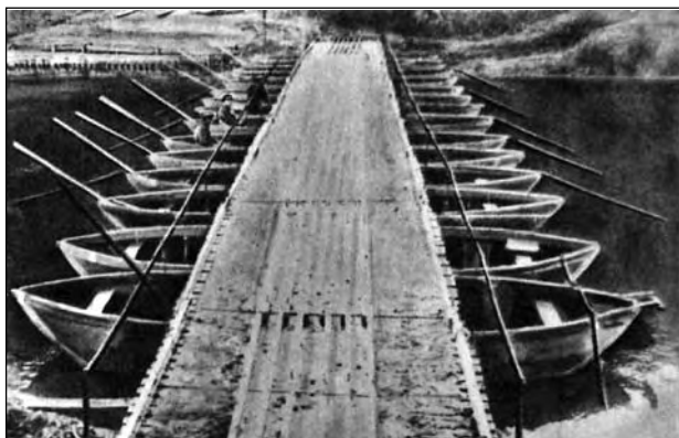
Наплавной мост из принятого на вооружение в 1932 году нового понтонного парка НЛП
